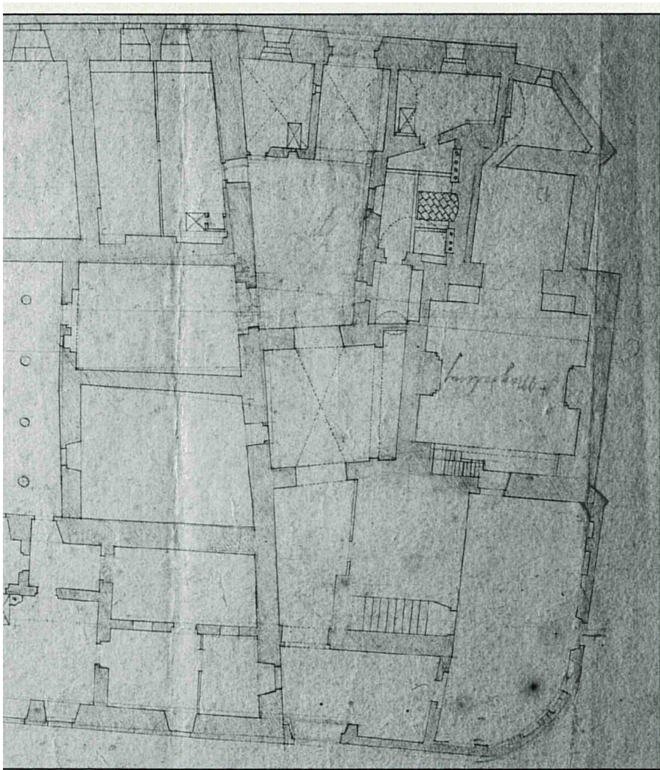
15. Najstarszy pomiar kościoła Św. Marii Magdaleny, z początku wieku XIX. Reprodukacja w publikacji Sroka, Szyma, Betlej, Dworzak, Bałus 2015. Kościół po prawej (napis odwrócony), po lewej Collegium Iuridicum, między nimi Dom Kanoniczy przy ulicy Grodzkiej (zob. il. 18).
