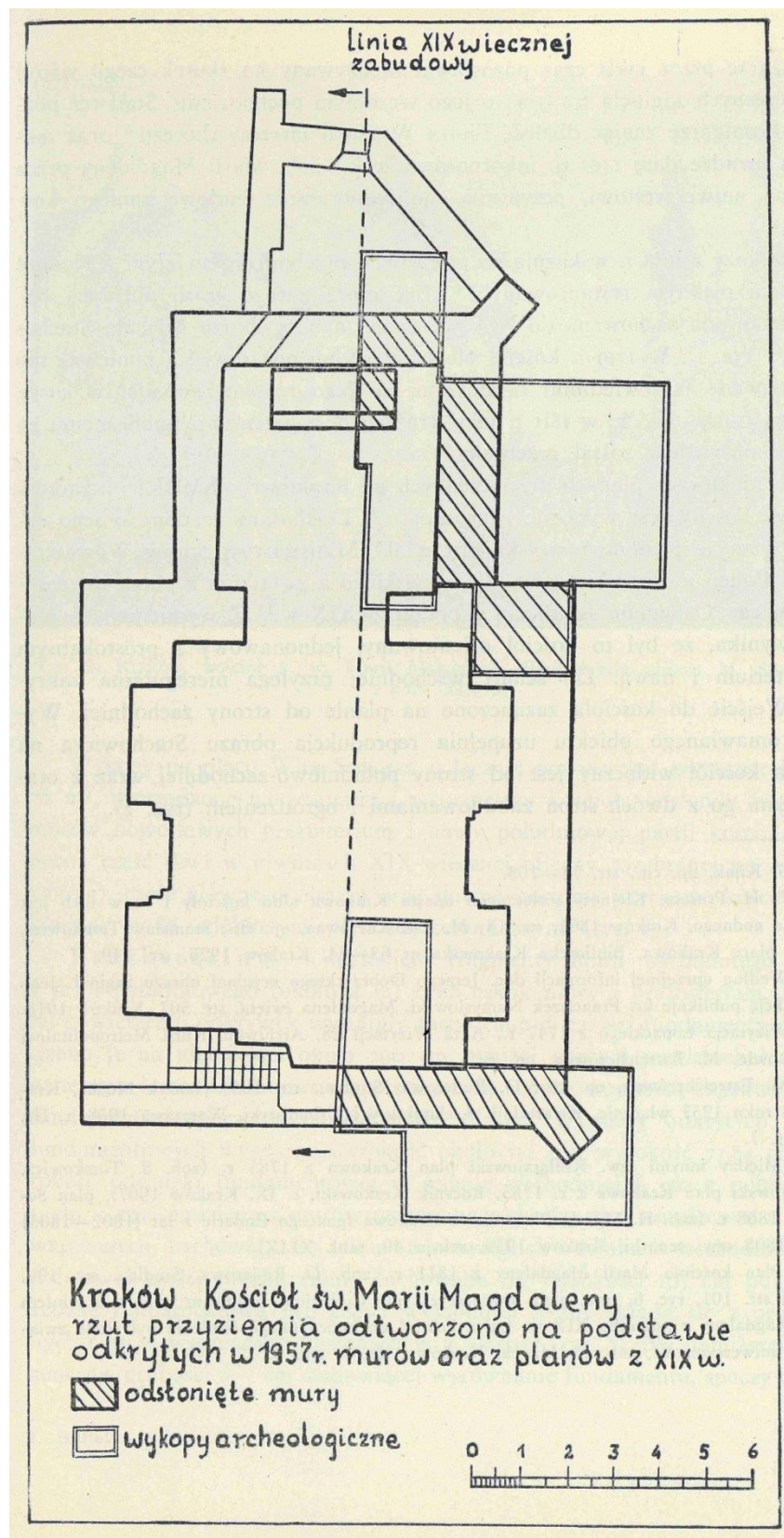
9. Dokumentacja pozostałości kościoła Św. Marii Magdaleny i rekonstrukcja stanu pierwotnego. Rysunek w publikacji Lenkiewicz 1959, ryc. 1.
