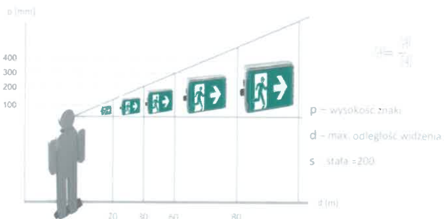
Rysunek 7 | Znaki oświetlone wewnętrznie (stała s = 200)
