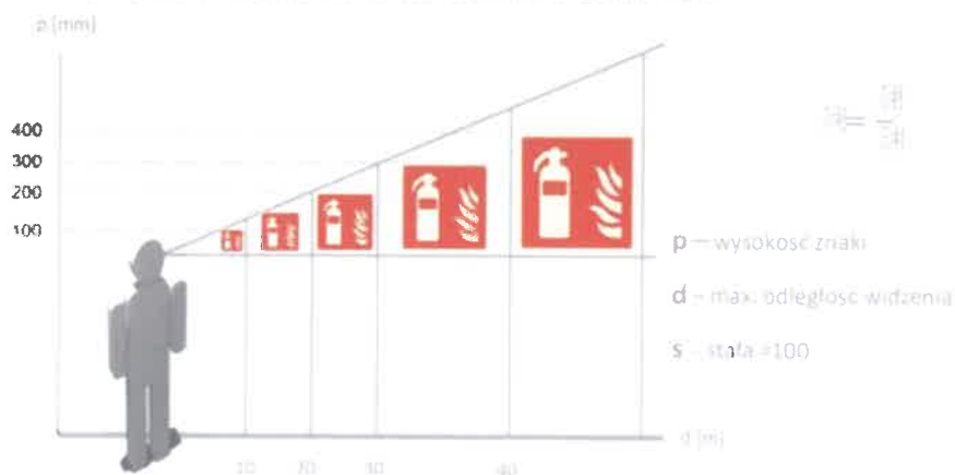
Rysunek 6 | Znak przeciwpożarowy (stała s = 100)
