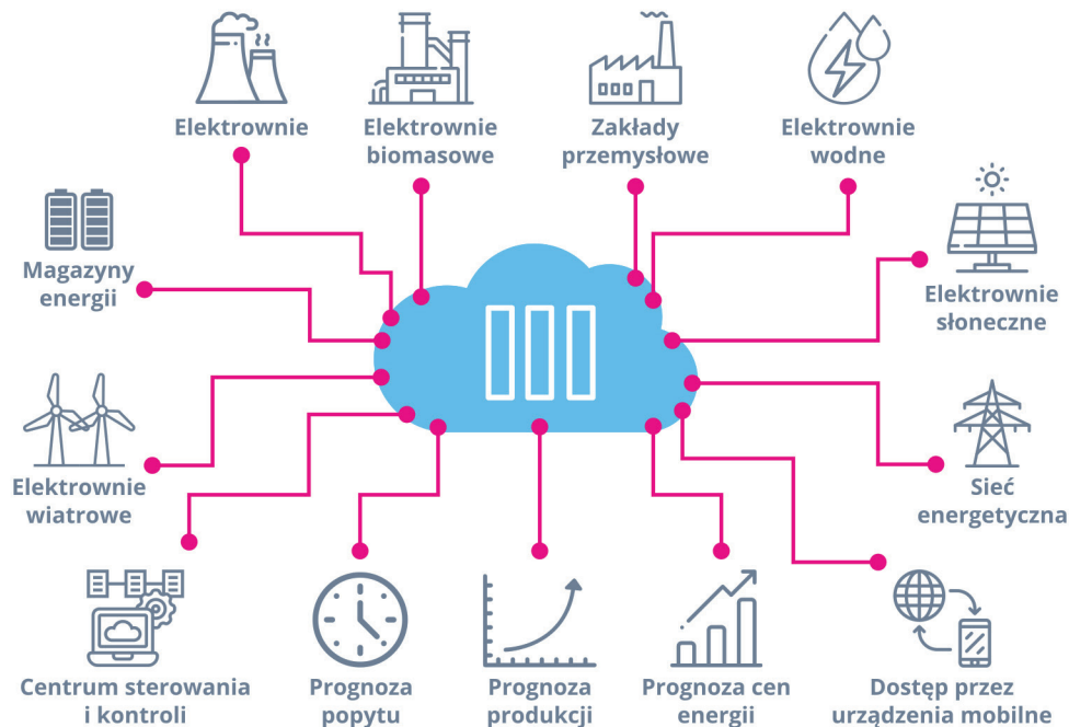
Rysunek 6: Elektrownia wirtualna (wg ABB)
