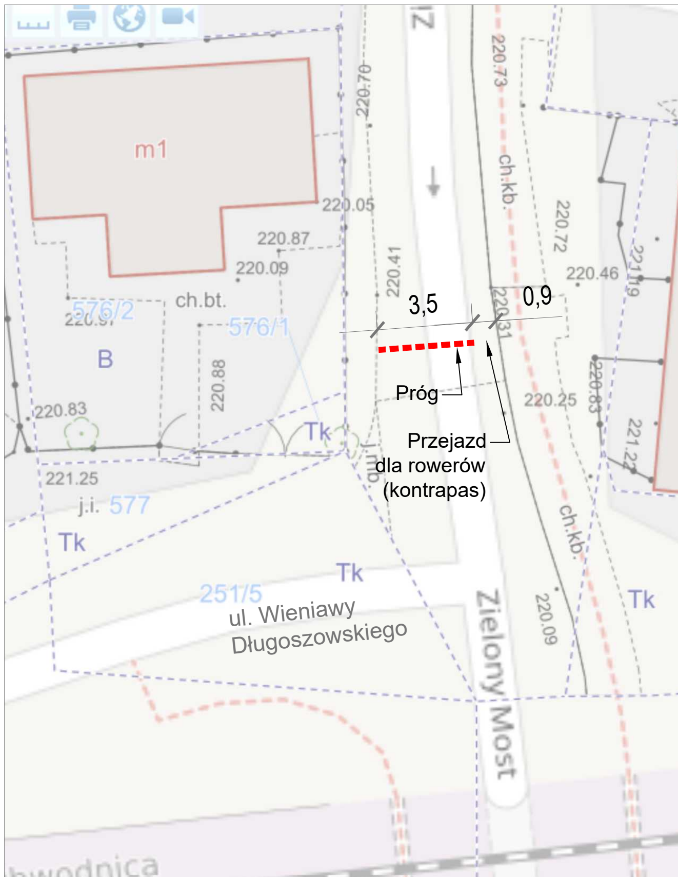
Zał. 1 Orientacyjna lokalizacja progu zwalniającego
